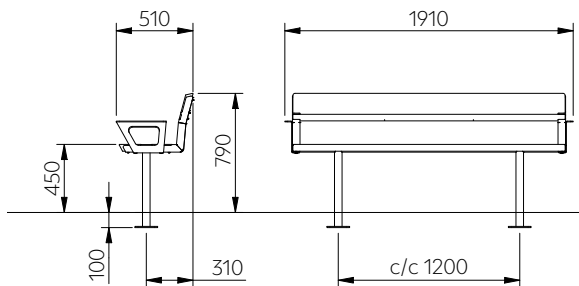
DAG110
