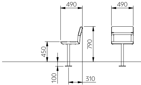
DAG200 DAG300 (360°∞)
