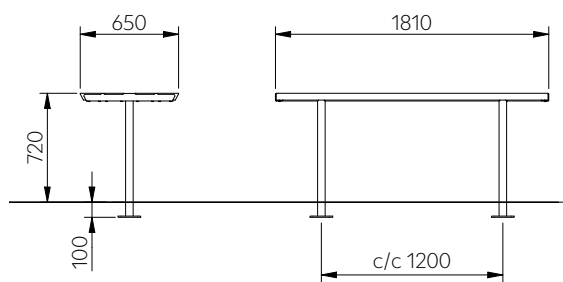
DAG700
