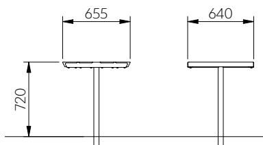
DAG600
