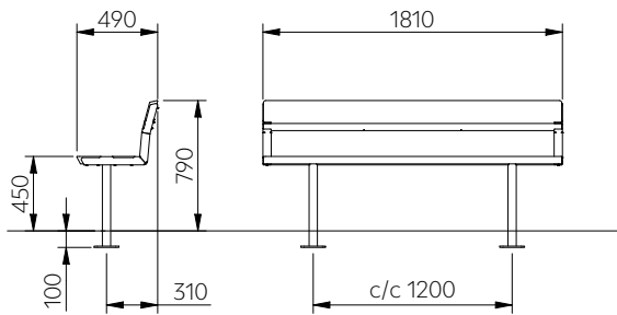
DAG100
