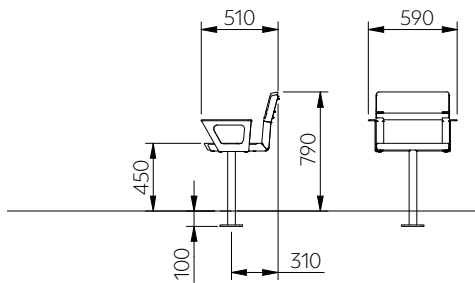
DAG210 DAG310 (360°∞)
