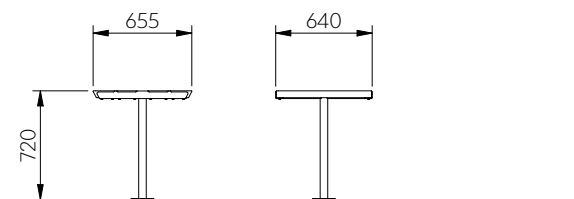
DAG601
