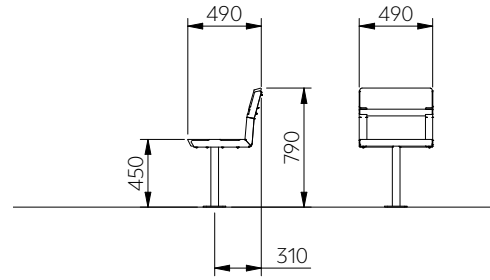
DAG201 DAG301 (360°∞)
