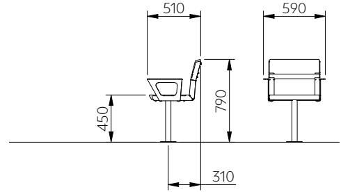
DAG211 DAG311 (360°∞)
