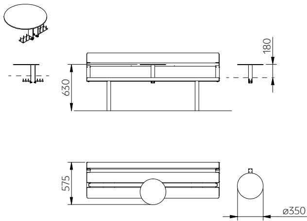
DAG035
