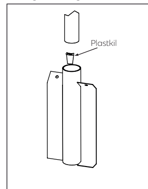
Nedgrävningssfundament 48/76
