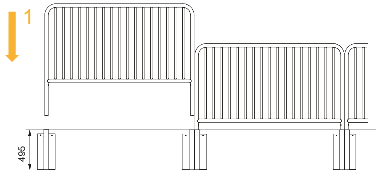
Nedgrävningsfundament 48
