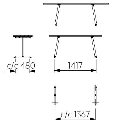
Fastsättning i marknivå
